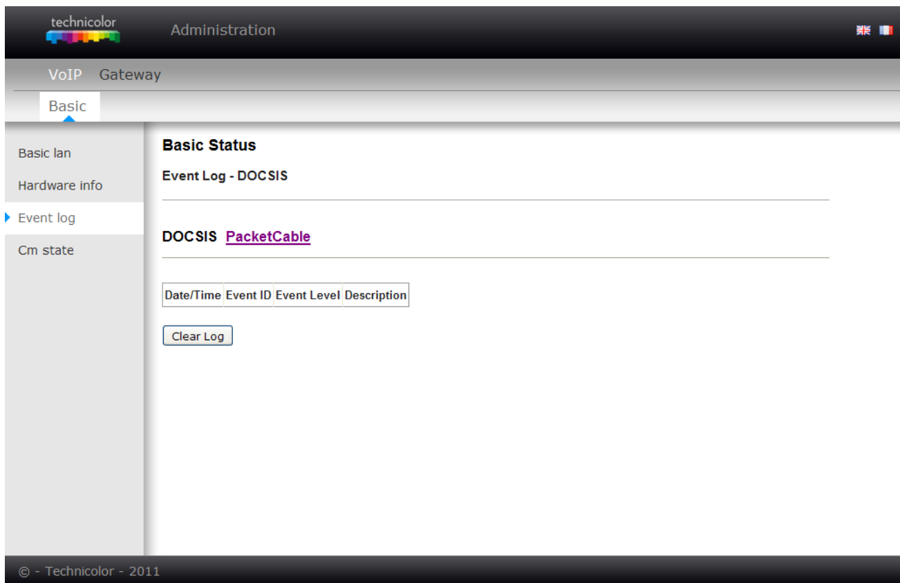
Fig. 2-47 VoIP\Basic\Event log\DOCSIS
